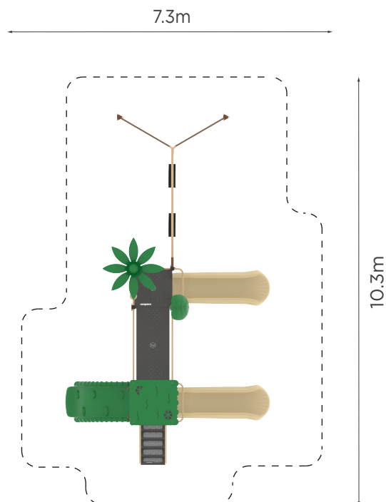
Vista superior:
